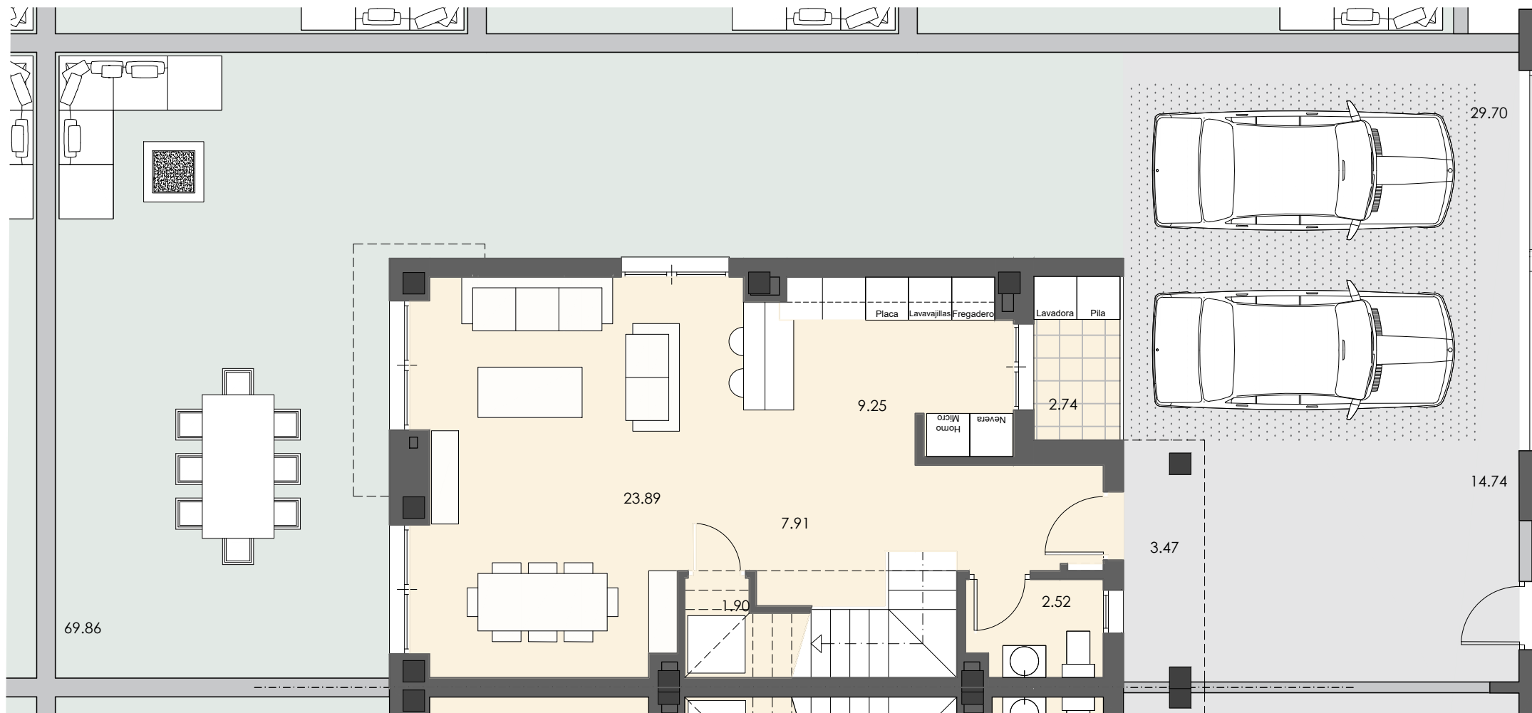
PLANTA BAJA
